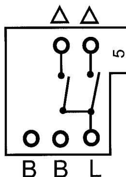
Kopplingsschema
